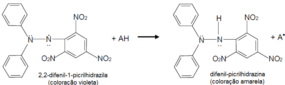
Figura 12. Esquema de mecanismo de redução do radical livre DPPH. Fonte: Os autores.
