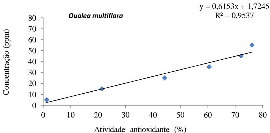
Figura 23. Curva de calibração obtida no ensaio pelo método \beta -caroteno/ácido linoleico no comprimento de onda 470 nm. Fonte: Os autores.
