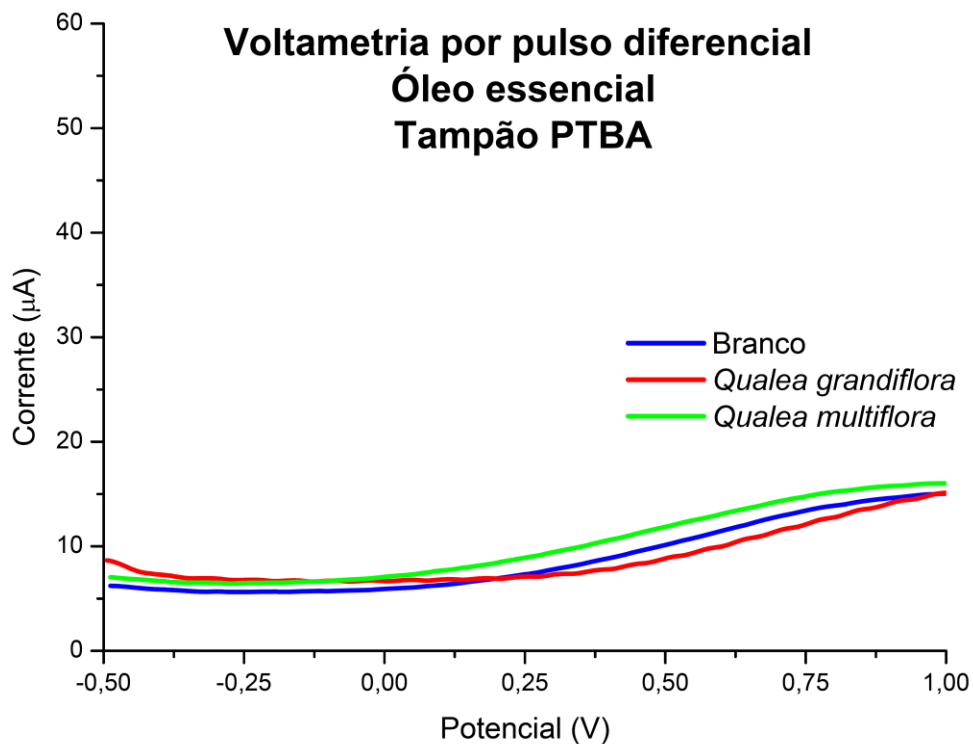
Figura 22. Amostra do extrato diluída em etanol com concentração de 2000 \mu\text{g.mL} , com tampão de perclorato de tetrabutilamônio. Fonte: Os autores.
