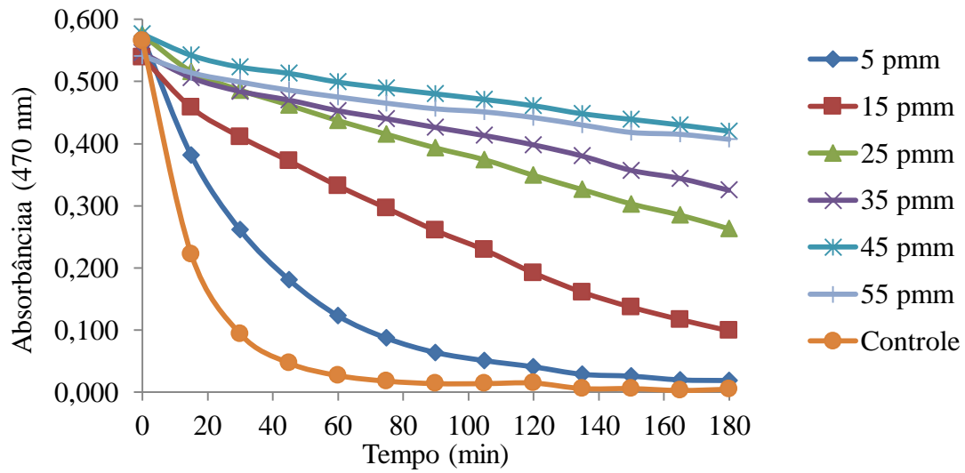
Figura 24. Atividade antioxidante do extrato etanólico de Qualea multiflora pelo método \beta -caroteno/ácido linoleico. Fonte: Os autores.
