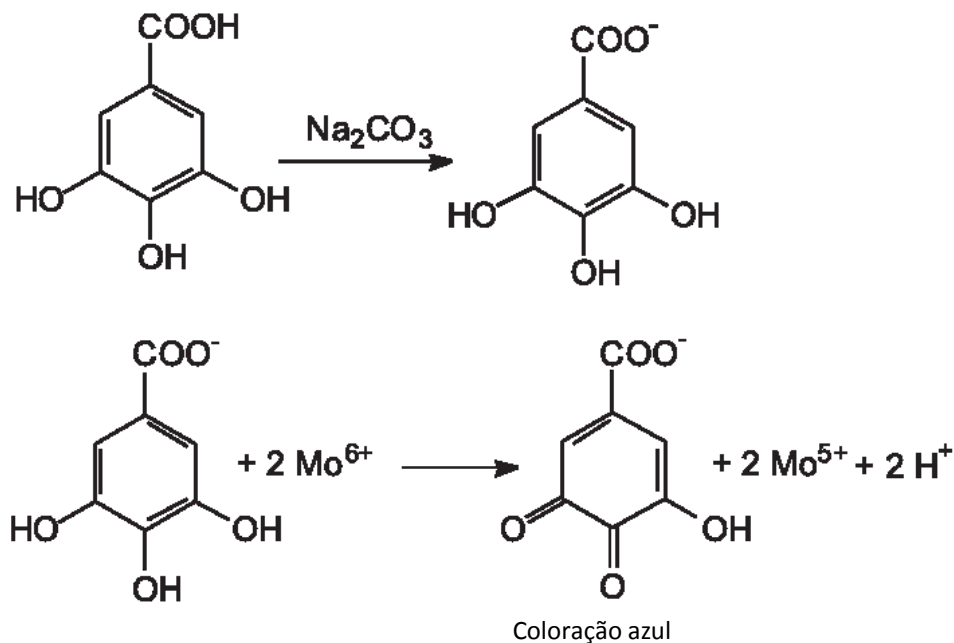
Figura 14. Reação do ácido gálico e a formação do complexo com molibdênio. Fonte: Oliveira et al. (2009).
