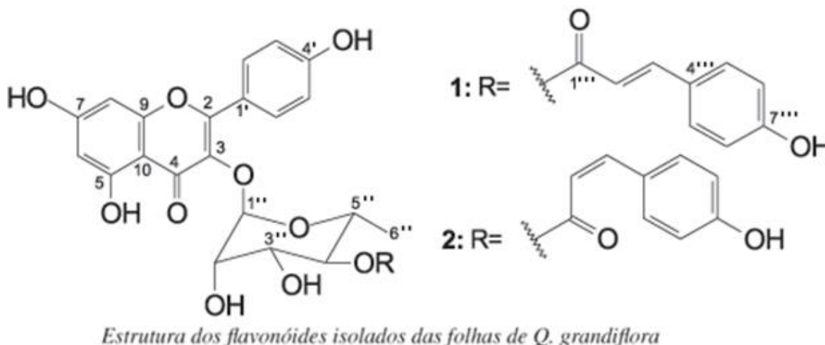
Figura 4. Estrutura de flavonoides isolados de extrato etanólico de folhas de Qualea grandiflora . Fonte: Os autores.
