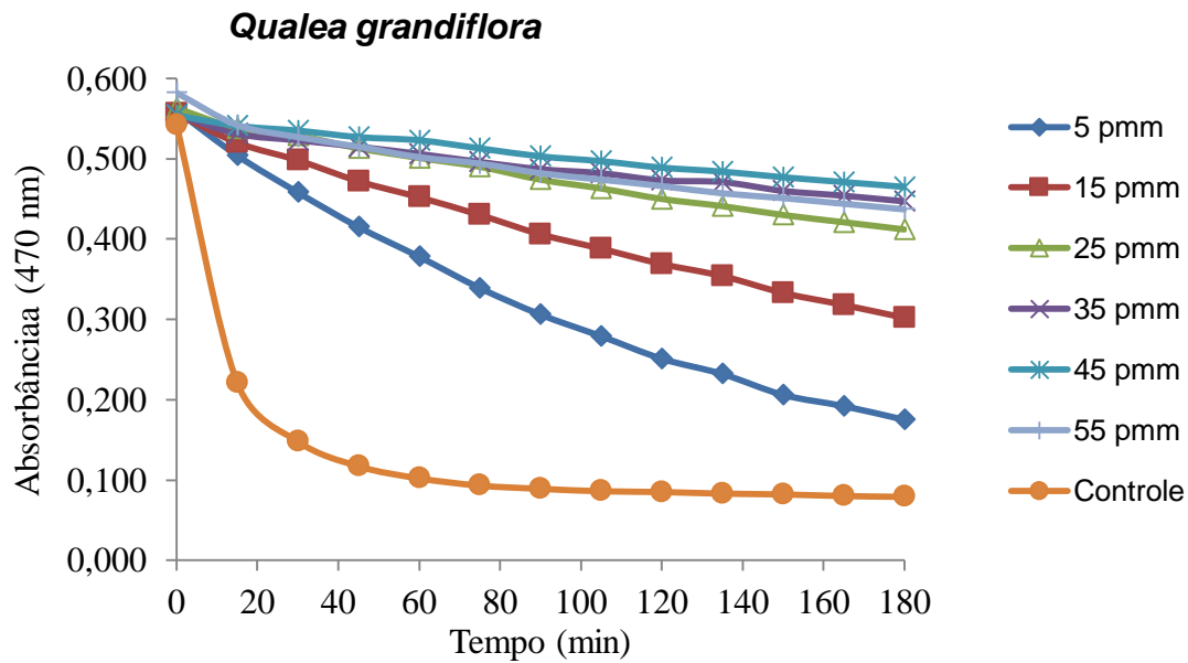
Figura 26. Atividade antioxidante do extrato etanólico de Qualea grandiflora pelo método \beta -caroteno/ácido linoleico. Fonte: Os autores.
