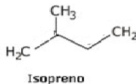
Figura 9. Esquema de unidade de isoprenóides. Fonte: Os autores.
