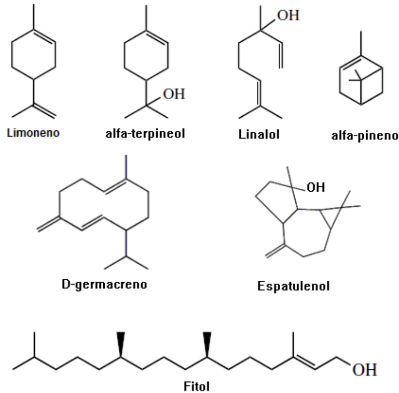
Figura 10. Estrutura de Monoterpenos, sesquiterpenos e diterpenos identificados em plantas do Cerrado. Fonte: Cunha et al. (2013), Londe (2004), Martins (2012) e Rocha (2011).
