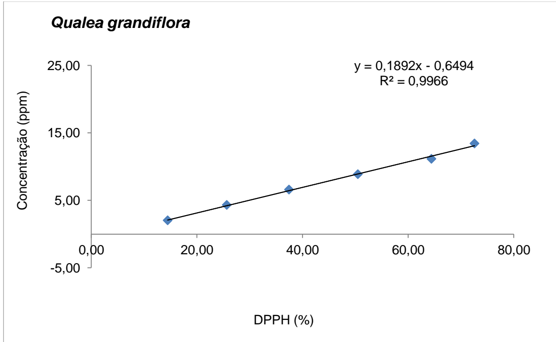
Figura 27. Concentração (ppm) dos extratos etanólicos de Qualea grandiflora em função da porcentagem de DPPH. Fonte: Os autores.
