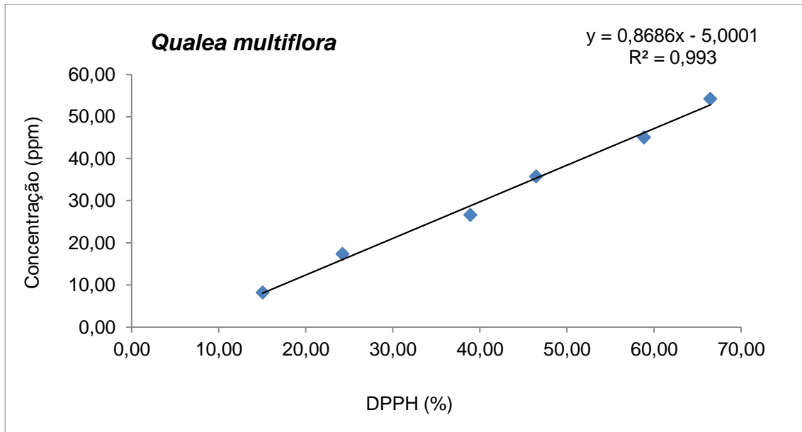
Figura 28. Concentração (ppm) dos extratos etanólicos de Qualea multiflora em função da porcentagem DPPH. Fonte: Os autores.
