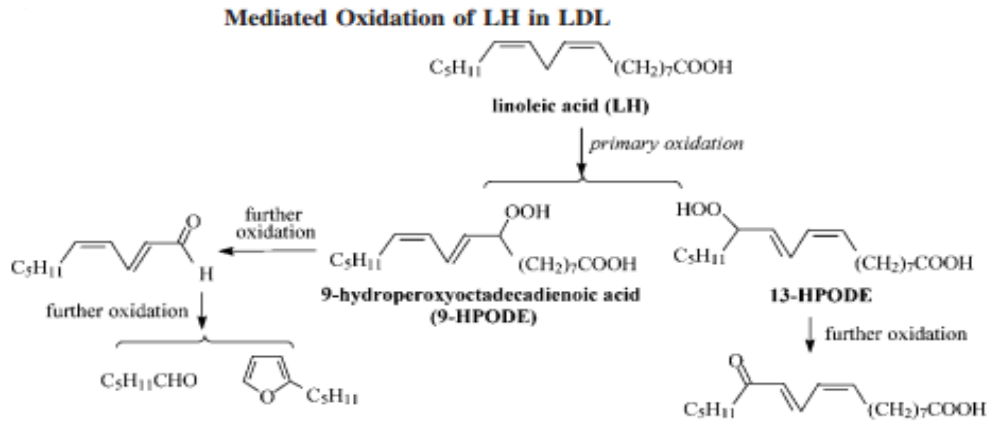
Figura 13. Esquema da oxidação do ácido linoleico. Fonte: Liu (2010).
