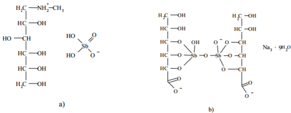
Medicamentos usados atualmente contra a leishmaniose; a) antimoniato de meglumine e b) estibogluconato de sódio.
