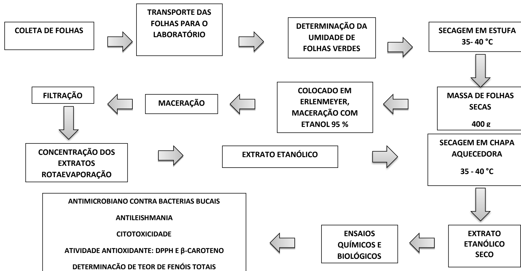
Figura 16. Fluxograma do preparo e obtenção do extrato etanólico a partir de amostras de folhas. Fonte: Os autores.
