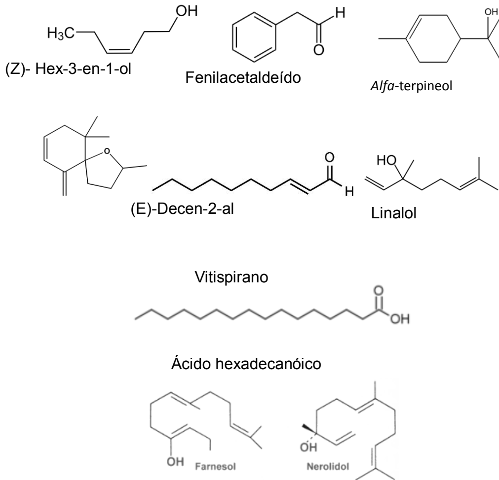
Figura 20. Esquema de alguns compostos do óleo essencial de folhas de Q. grandiflora e Q. multiflora . Fonte: Os autores.
