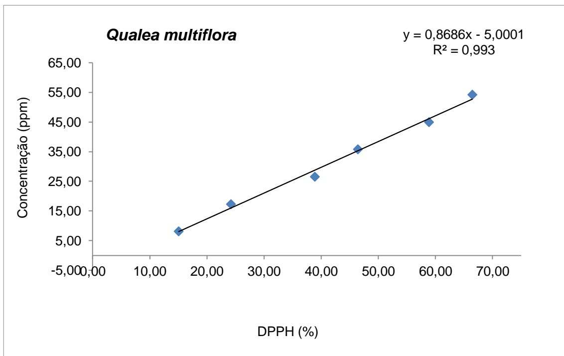
Figura 25. Curva de calibração obtida no ensaio pelo método \beta -caroteno/ácido linoleico no comprimento de onda 470 nm. Fonte: Os autores.
