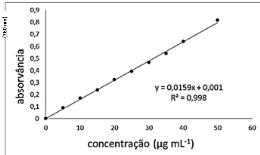
Figura 29. Curva de calibração do ensaio Fenóis Totais. Fonte: Os autores.
